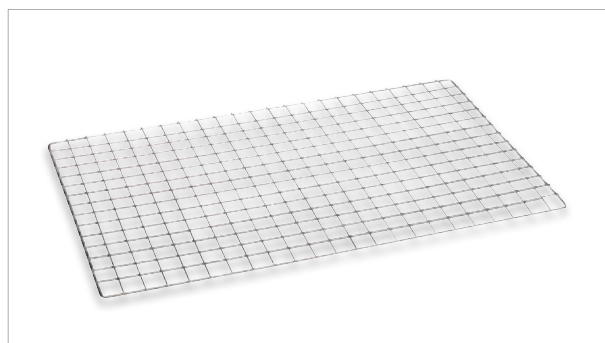
Trådshylde, 600 x 400 mm Maskestørrelse ca. 22,5 x 23,0 mm Til brug på teleskopskinner bestilles i stedet varenr. 2264502/01.
